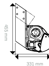
Montage tegen de dakspanten dakspantconsoles*
