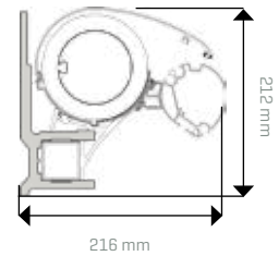
Montage tegen de wand muurconsole s
