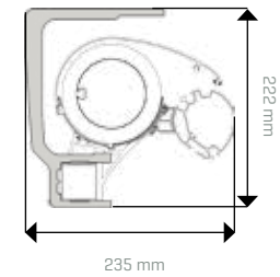
Montage tegen de dakspanten dakspantconsole s*
