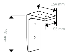
Montage tegen het plafond plafondbeugels*
