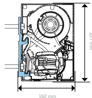
Montage tegen de wand muurconsole s
