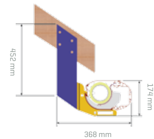
Montage tegen de dakspanten dakspantconsoles*
