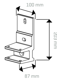
Montage tegen de wand muurconsole
