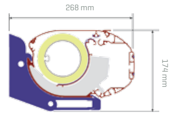
Montage tegen de wand muurconsoles
