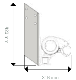
Montage tegen de dakspanten dakspantconsole s*
